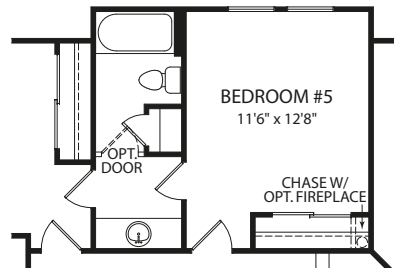
Optional Bedroom #5
