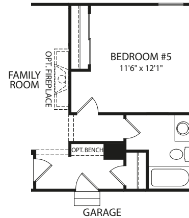
Optional Bedroom #5
