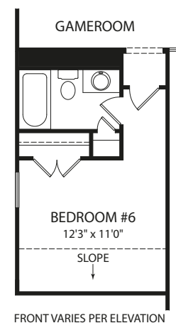
Optional Bedroom #6
