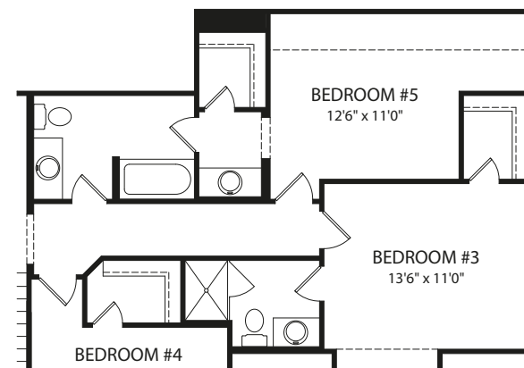
Optional Bedroom #5
